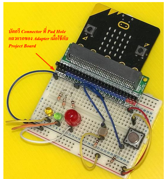
รูปการประยุกต์ใช้งานร่วมกับ Project Board
