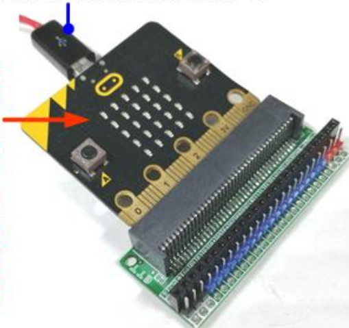
รูปการต่อใช้งาน Adapter กับบอร์ด micro: bit
