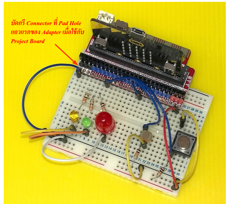
รูปการประยุกต์ใช้งานร่วมกับ Project Board
