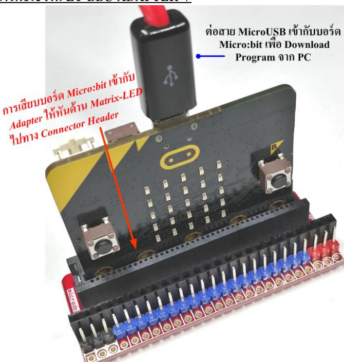
รูปการต่อใช้งาน Adapter กับบอร์ด micro:bit
