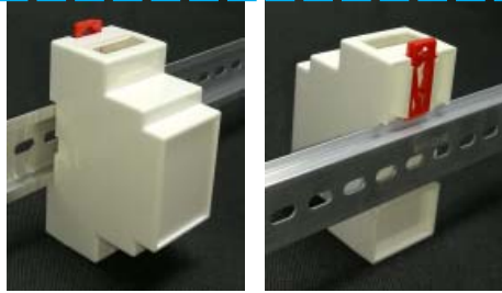
• รูปกล่องเมื่อติดตั้งบนราง DIN 35 mm.
